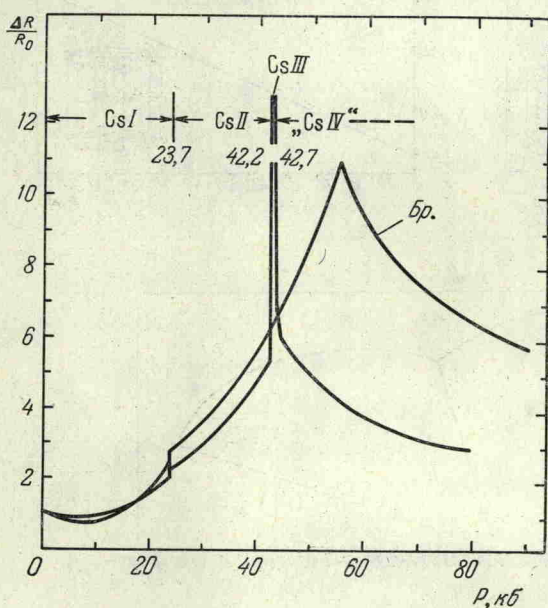
Рис. 2. Зависимость электросопротивления Cs от давления (по работе 22 ).
